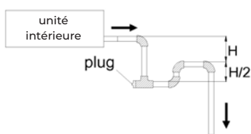
Figure 6.5 Drainage de la tuyauterie pièges à eau
