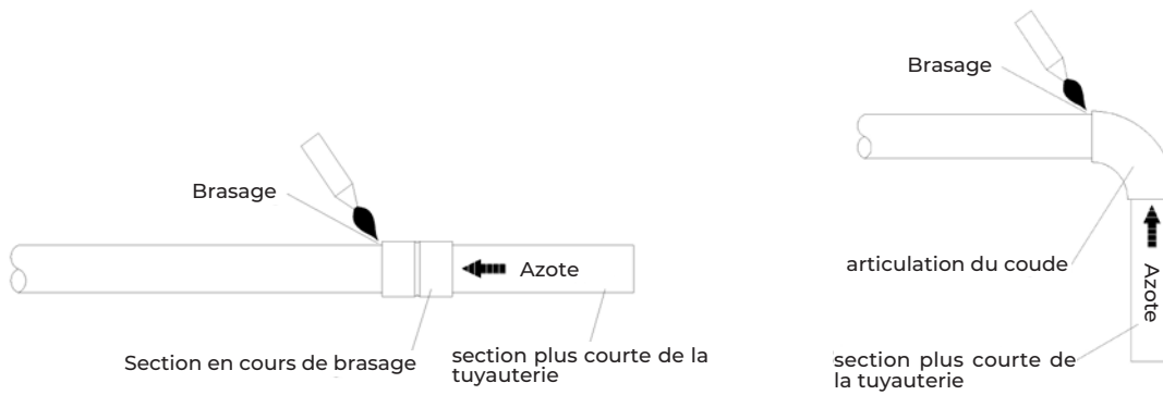
Figure 5.5 Flux d'azote du côté le plus court pendant le brasage
