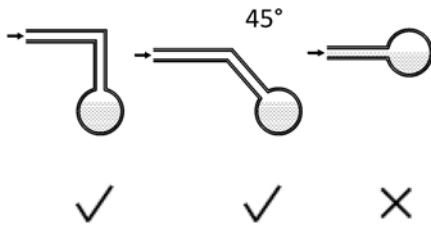
Figure 6.3 Tuyauterie d'évacuation secondaire rejoignant la tuyauterie d'évacuation principale
