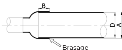
Figure 5.7 Chevauchement et espacement des tuyauteries pour les joints brasés
