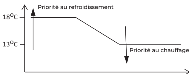
Figure 11.2 Mode priorité automatique
