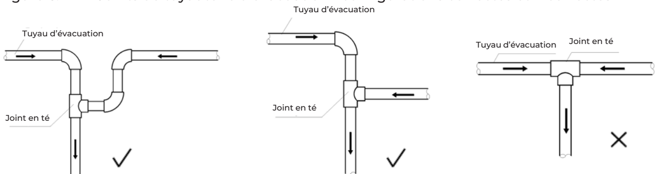
Figure 6.2 Joints de tuyauterie d'évacuation - configurations correctes et incorrectes
