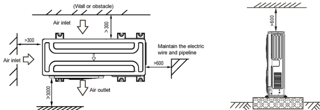
Figure 3.1 Installation d'une seule unité (unité : mm)
