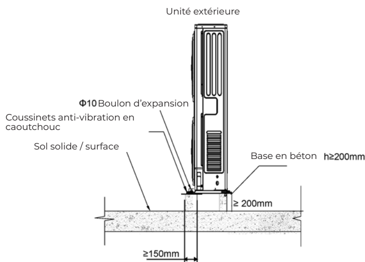
Figure 3.4 Structure type de la base en béton de l'unité extérieure (unité : mm)
