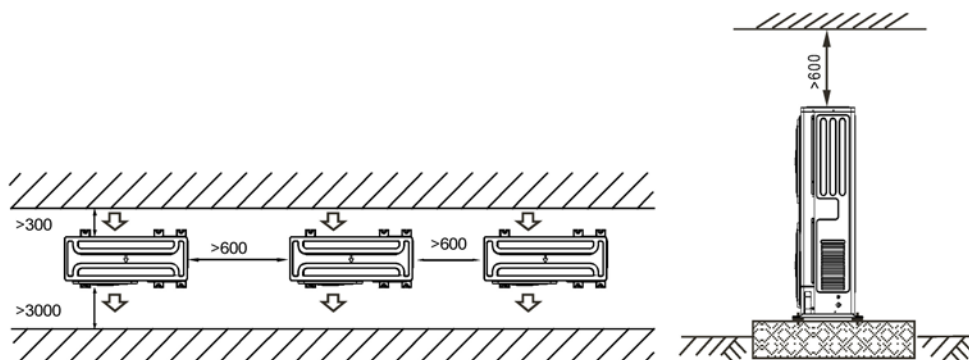
Figure 3.2 Raccordement parallèle des deux unités ou plus (unité : mm)
