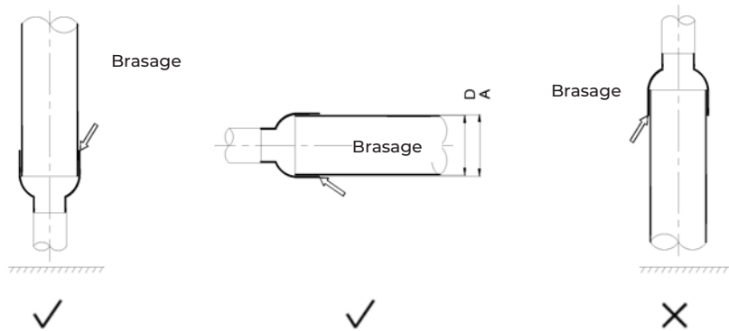
Figure 5.6 Orientation de la tuyauterie pendant le brasage
