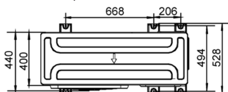
Figure 3.5 Positionnement et espacement du boulon d'expansion (unité : mm)
