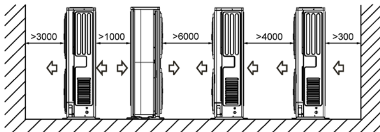
Figure 3.3 Liaison parallèle entre l'avant et l'arrière (unité : mm)
