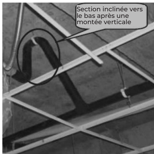
Figure 6.6 Section inclinée vers le bas de la tuyauterie d'évacuation
